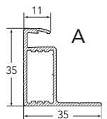
Rahmenquerschnitt A
